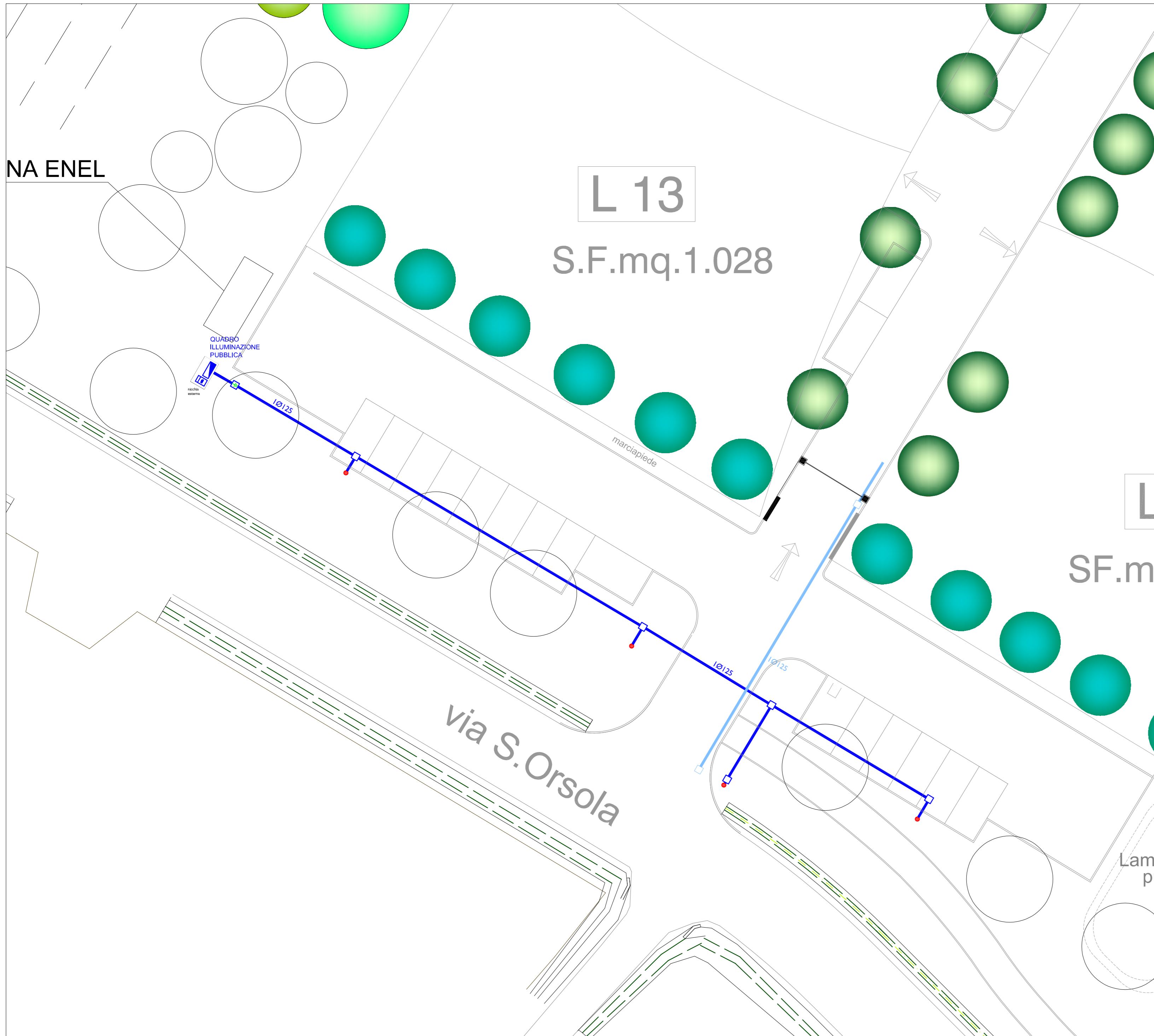
PLANIMETRIA OPERE EDILI - SCALA 1:200
