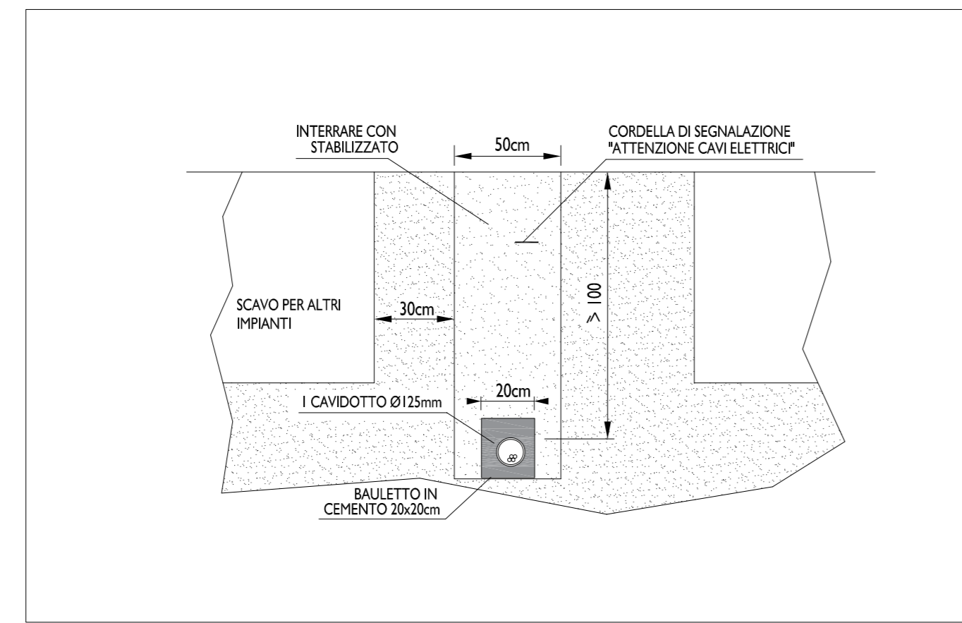
PARTICOLARE SCAVO ILLUMINAZIONE SCALA 1:20
