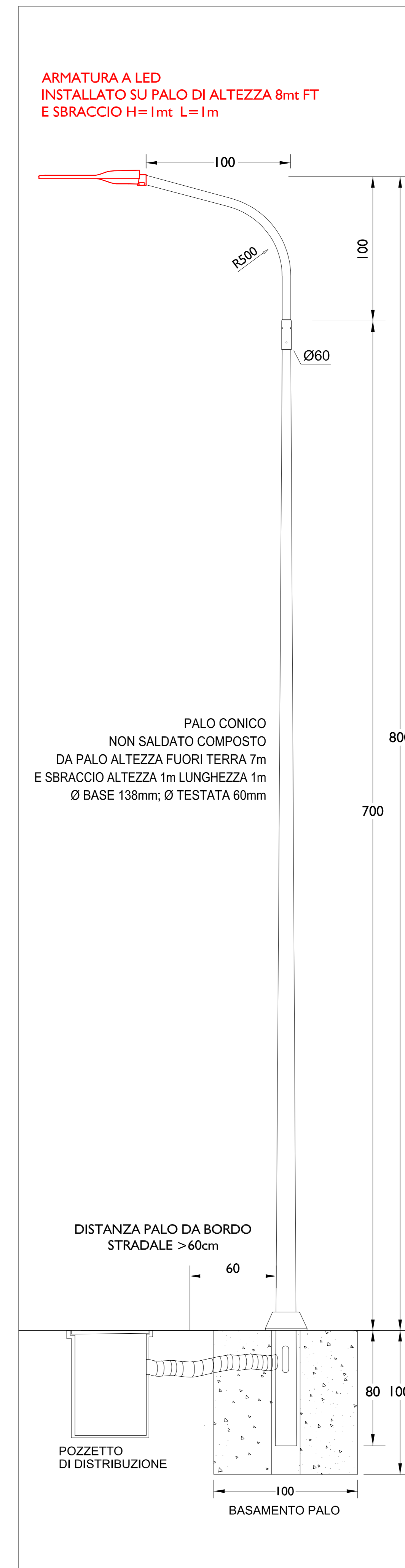
PARTICOLARE PALO - SCALA 1:20
