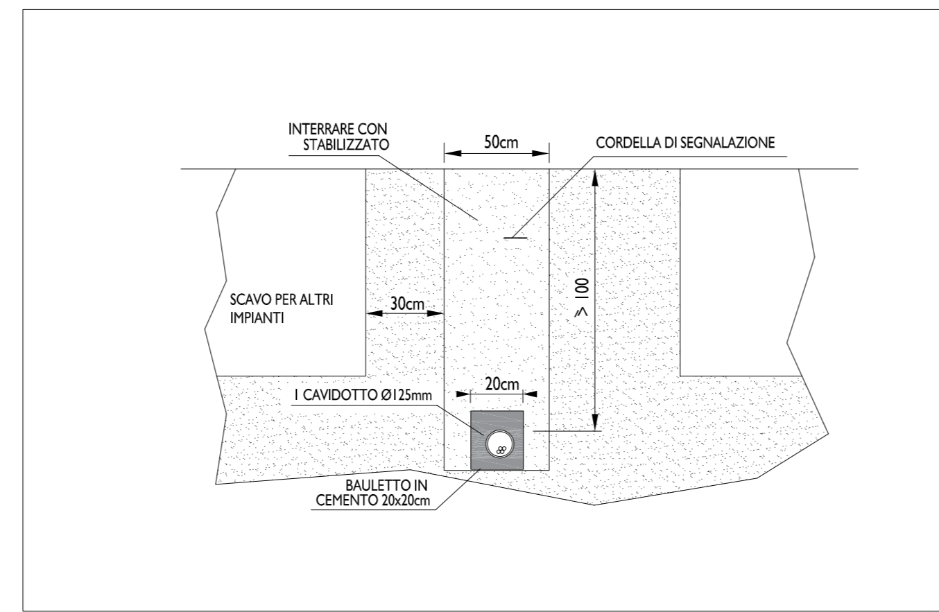
PARTICOLARE SCAVO RETE CABLAGGIO SCALA 1:20
