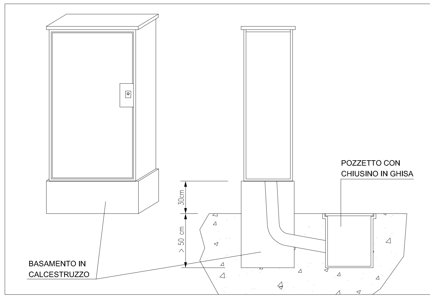
PARTICOLARE NICCHIA - SCALA 1:20
